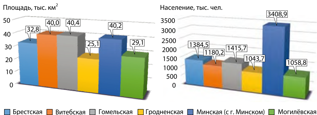
Рис. 5. Площадь (тыс. км 2 ) и население (тыс. чел.) областей Беларуси на 01.01.2018
